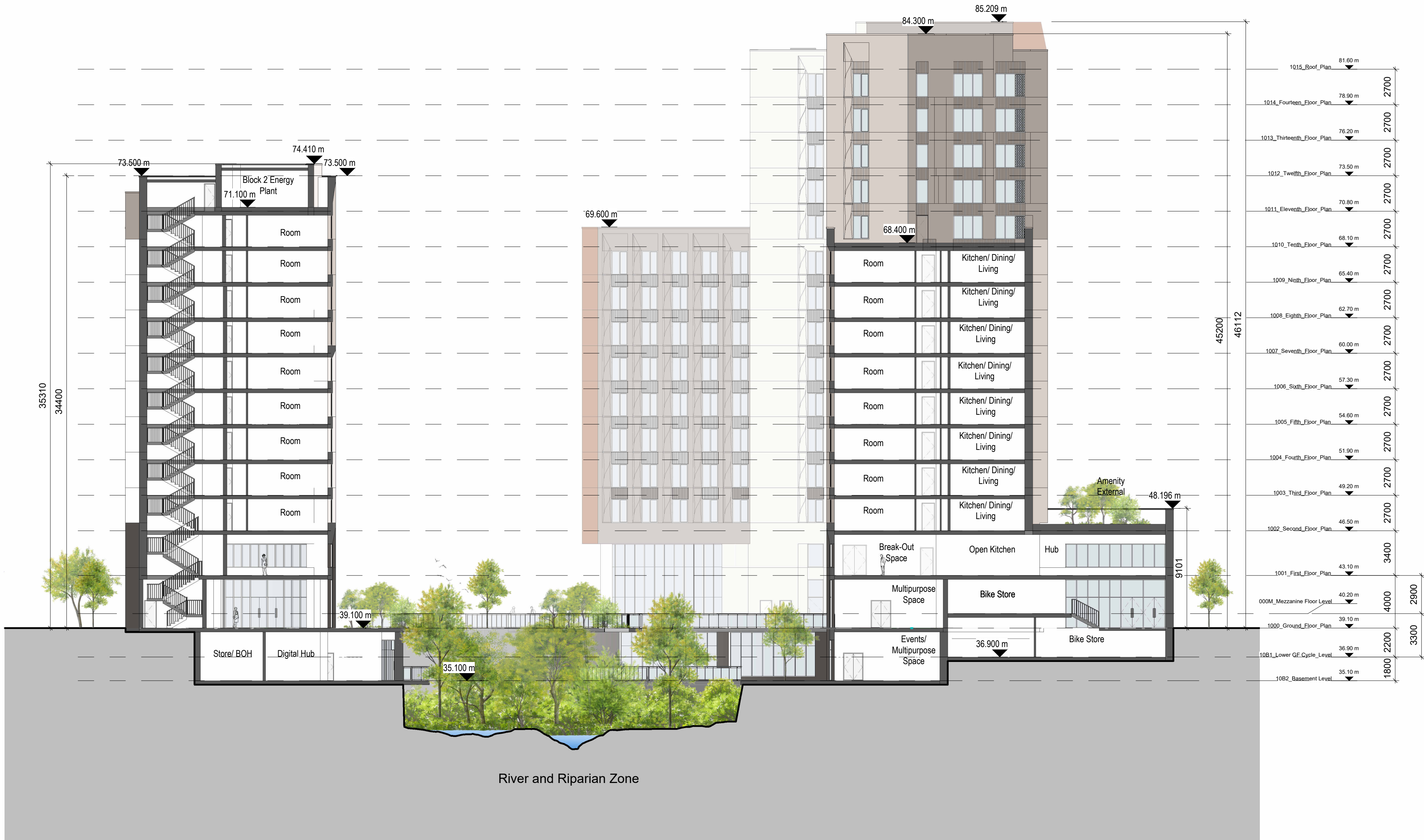
1 Section BB 1 : 200
